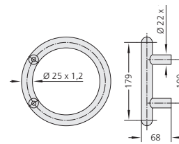
Type ER-25.R
